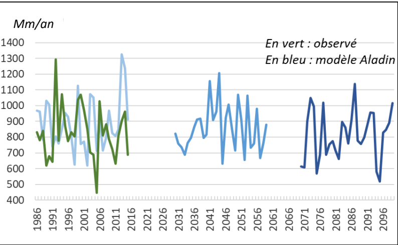
Évolution annuelle de la pluviométrie (modèle Aladin)
